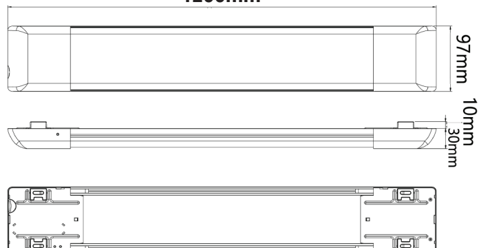
BATTENS001 - BACK
